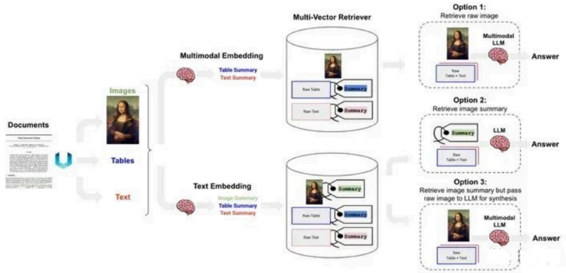
图6 多模态RAG
